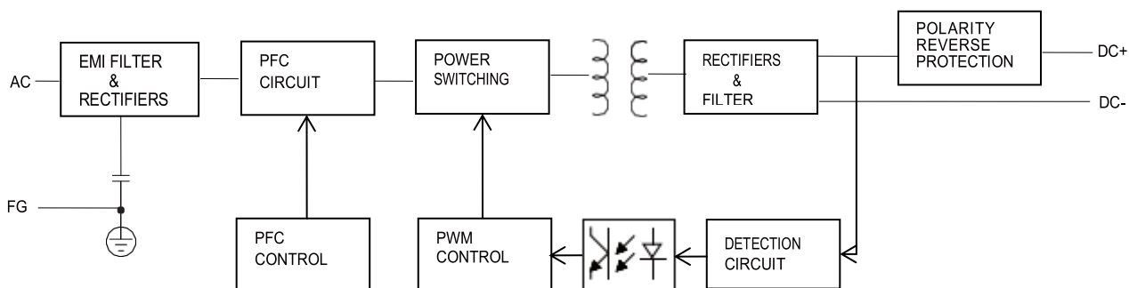
■ 原理框图
